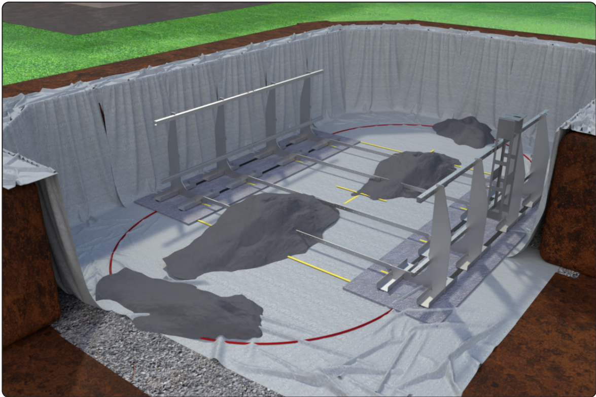
Splitt in die Grube einbringen
