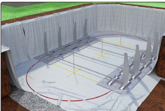
Zugstreben montiert
