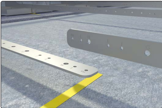
Zugstreben auslegen. (Montage außerhalb der Baugrube)
