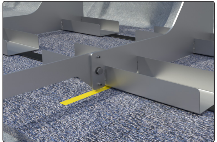
Zugstreben an L - Träger montiert
