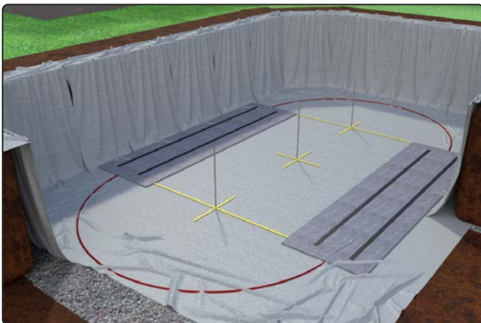
Vierkantrohre platziert und plan abgezogen
