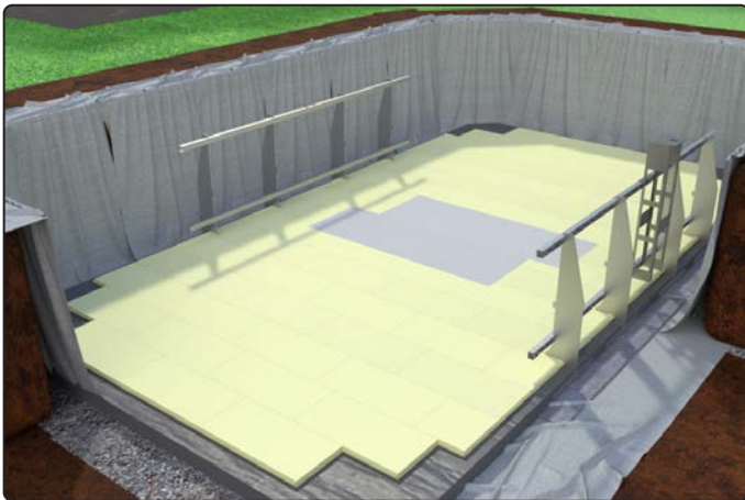
Vinylplatten aus der Mitte im Versatz verlegen
