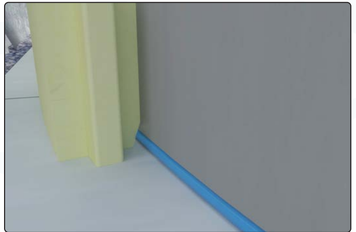
Rundschalung an der Bodenschiene 45° ansträgen
