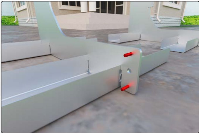
Spannhülsen einschlagen (Montage außerhalb Baugrube)
