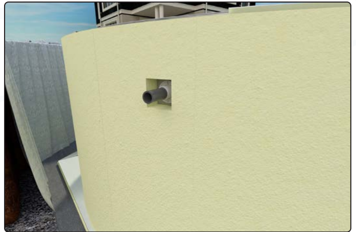
Einbauteile ausschneiden
