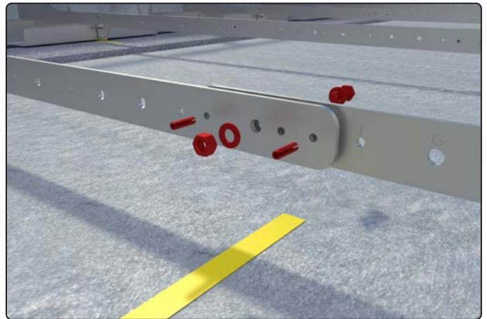
Zugstreben mit Schraube und Spannhülsen verbinden. (Montage außerhalb der Baugrube)
