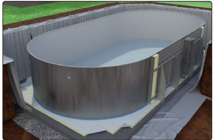
ca. 1cm Wasser einfüllen, Bodenfallen glätten
