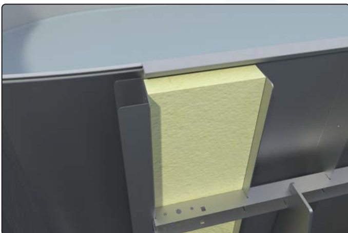
gerade Elemente des Handlaufs auf länge U-Bleche kürzen
