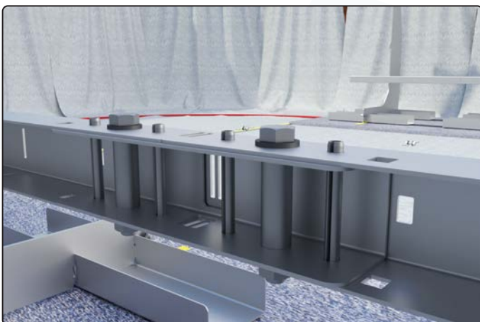
Querträgerverbinder mit Querträgern verbunden
