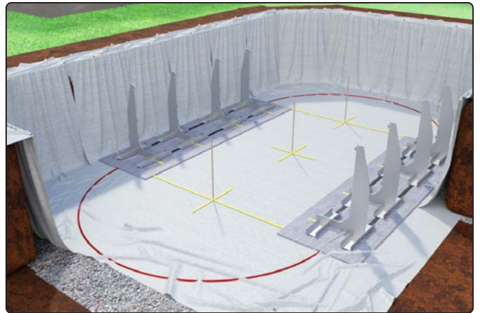
L - Träger grob positionieren
