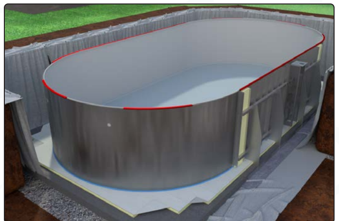
Handlaufsegmente aufstecken und verbinden. Letztes Segment erst nach vollständiger Befüllung aufstecken und anpassen
