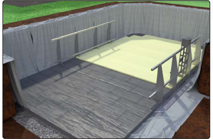
Bodenplatte mit Gesamtüberstand 30cm verlegen
