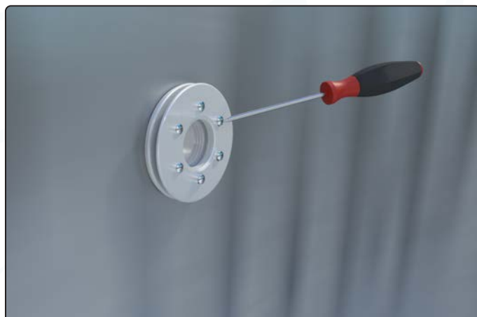
Flansch auf Grundkörper anschrauben
