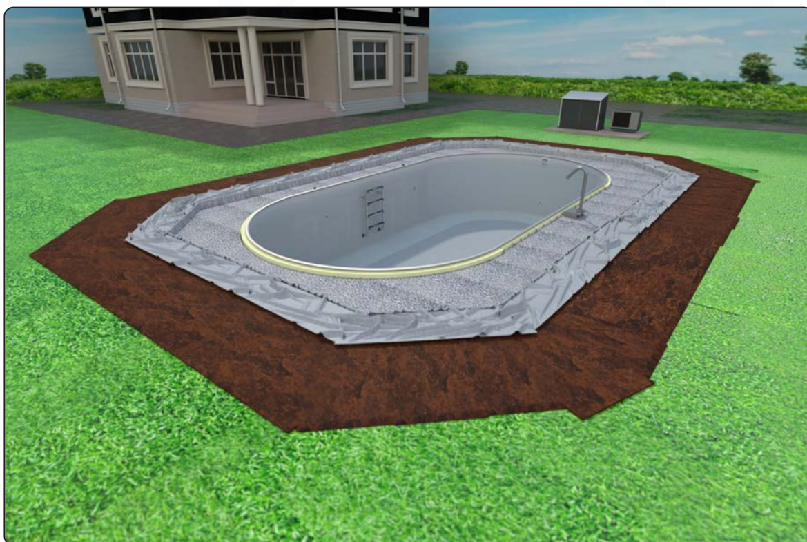
Baugrube gleichmäßig mit Kies aufgefüllt
