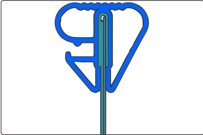
Querschnitt Handlauf mit Einhängesiege
