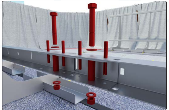
Explosionsansicht Querträgerverbinder
