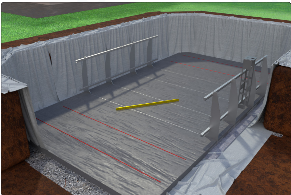
Mit einer langen Latte plan abziehen. Rohre (rot) dienen als weitere Abziehhilfe.
