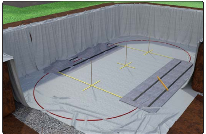
Vierkantrohre auf Höhe bringen, plan abziehen. Kies unter Vierkantrohre mit Hand stopfen.
