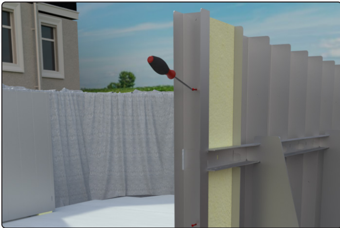
Abschlussprofile mit U-Blechen verschrauben
