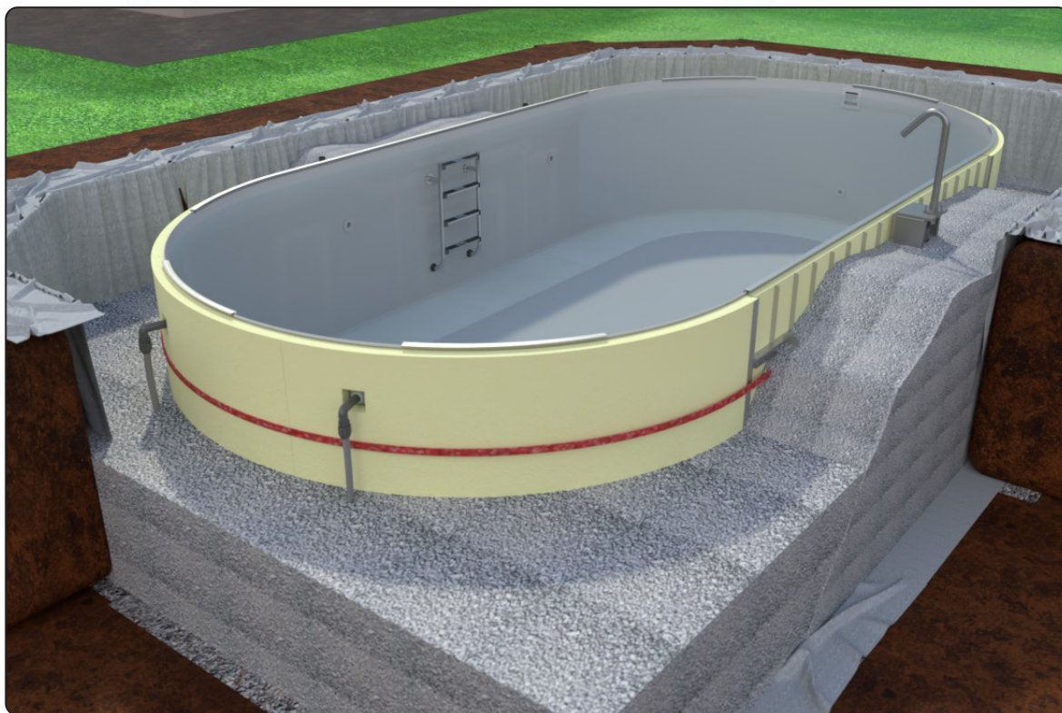
Kies gleichmäßig in die Baugrube einbringen
